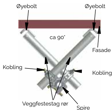
Eksempel på forankring som kan oppta horisontalkrefter
