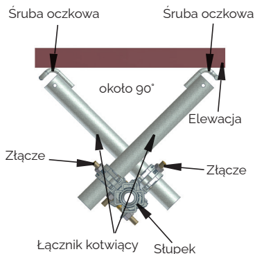
Przykład zakotwienia mogącego przenosić siły poziome
