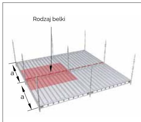
Rusztowanie Wolnostojące
