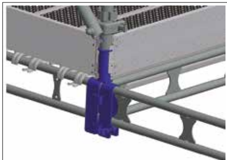
11. Uchwyt słupka dla podłużnicy
