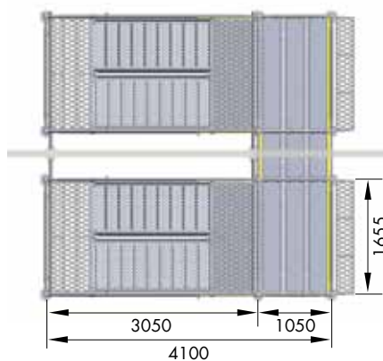
HAKI Trappetårn sammenbygd med et trappetårn på innsiden av bygget
